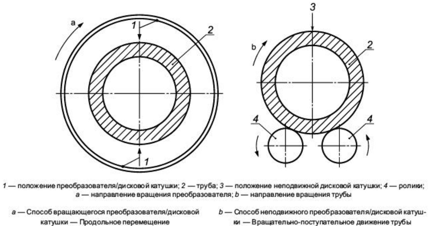
Рисунок 3 - Упрощенная схема вихретокового метода контроля с дисковой катушкой
