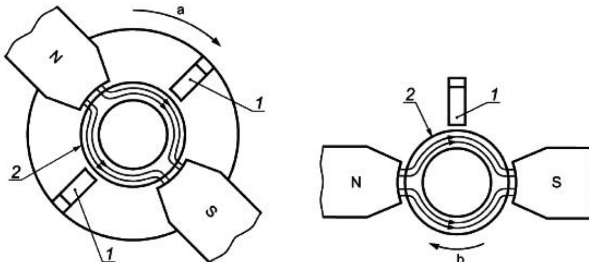
Рисунок 4 - Упрощенная схема определения продольных дефектов методом рассеяния магнитного потока
