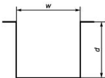
Рисунок 6 - Паз "N"- типа
