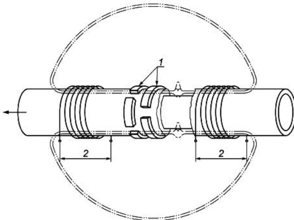
Рисунок 5 - Упрощенная схема определения поперечных дефектов методом рассеяния магнитного потока
